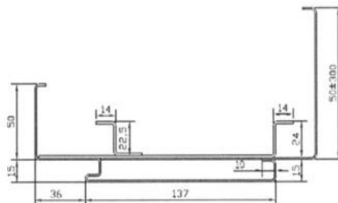
Przekrój ościeżnicy regulowanej z wyłożeniem. (zakres: 185-245; 245-305; 305-365)
