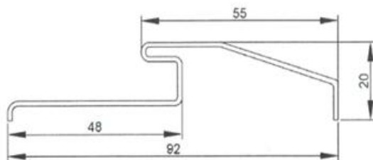
Próg stalowy
