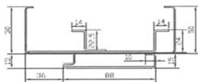
Przekrój ościeżnicy regulowanej. (zakres: 125-155; 155-185)
