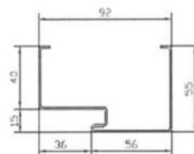
Przekrój ościeżnicy asymetrycznej
