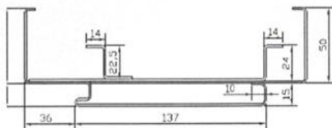
Przekrój ościeżnicy regulowanej. (zakres: 185-245; 245-305; 305-365)
