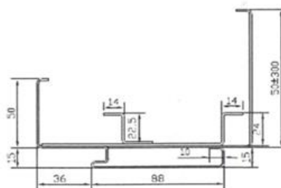
Przekrój ościeżnicy regulowanej z wyłożeniem. (zakres: 125-155; 155-185)
