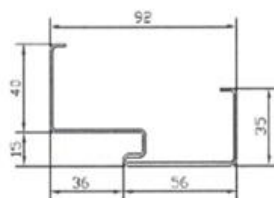
Przekrój ościeżnicy asymetrycznej
