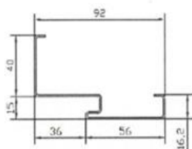
Przekrój ościeżnicy narożnej
